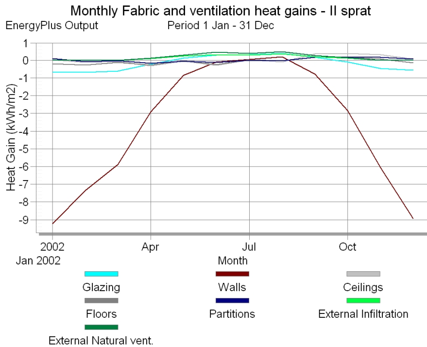
Slika 28. Mesečni spoljni dobici toplote za ceo stan
